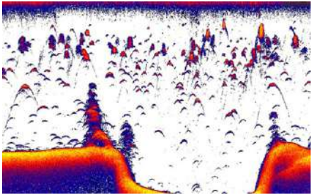
CHIRP 声呐
